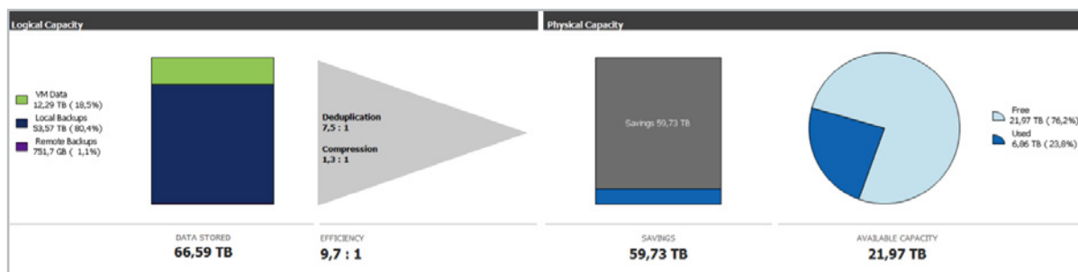
66,59 TB aan logische data gebruikt slechts 6,86 TB aan fysieke opslag
